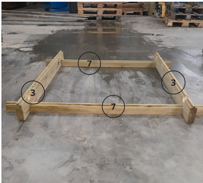
Osat 3 liitetään salvosliitoksistaan osien 7 päälle.
