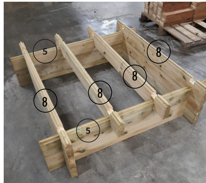
Liitetään osat 5 ja osat 8 kehikon päälle ja lisätään välituet osa 8.
