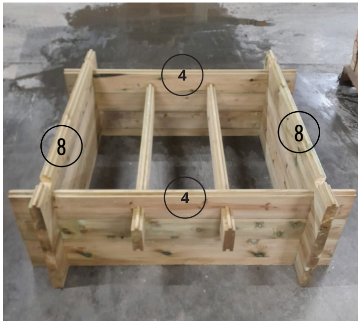
Liitetään osat 8 ja osat 4 kehikon päälle. Jatketaan arkun kokoamista osilla 8 sopivaan korkeuteen.
