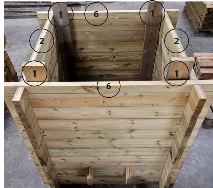
Viimeiseksi kerrokseksi liitetään osat 2 ja osat 6, sekä kiinnitetään läpipultein sidoslankut osa 1 kehikkoon. Loput pultit ja mutterit ovat kävelysillan kiinnitykseen sidoslankkuihin, sekä mahdollisten ankurointilenkkien kiinnitykseen.
